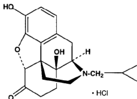
naltrexone hydrochloride
